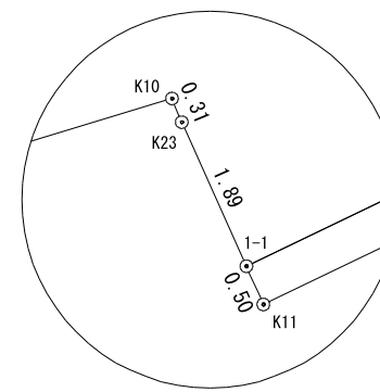
口部拡大図 1/100
