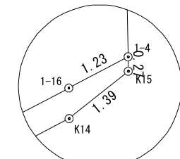
イ部拡大図 1/100
